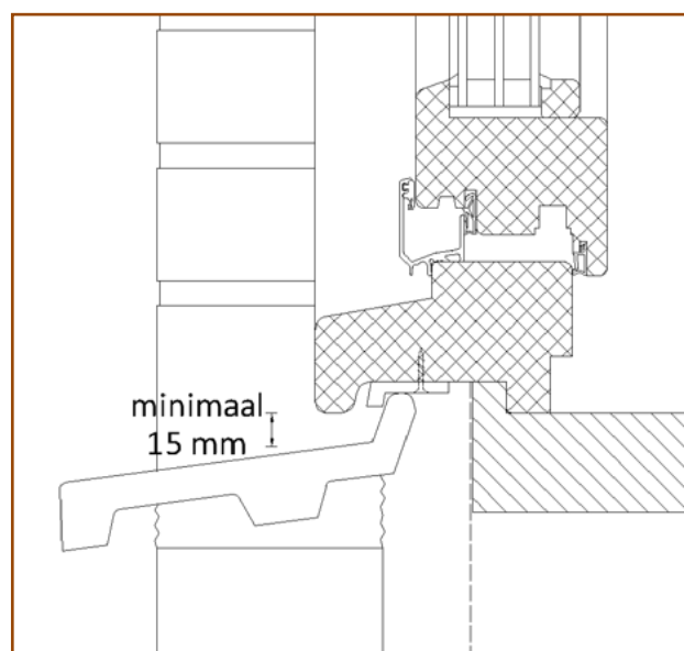
Figuur 6. Ruimte onder kozijn
