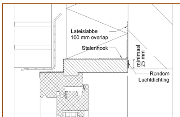
Figuur 4. Bovenaansluiting bij metselwerk
