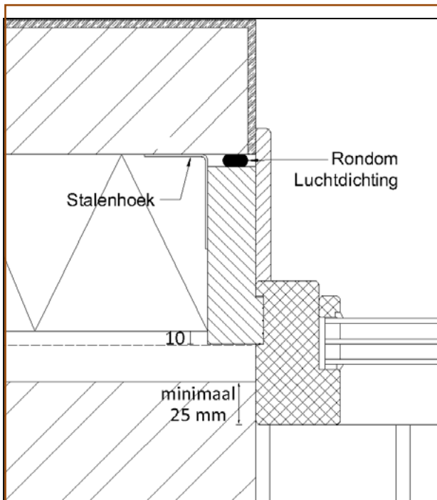
Figuur 7. Luchtdichting op gemetseld binnenblad
