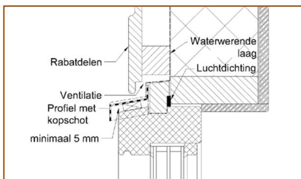
Figuur 5. Bovenaansluiting bij plaatgevel
